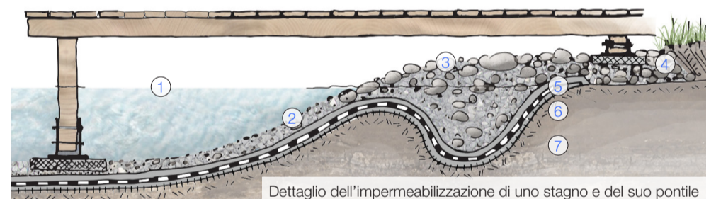
Dettaglio dell'impermeabilizzazione di uno stagno e del suo pontile
